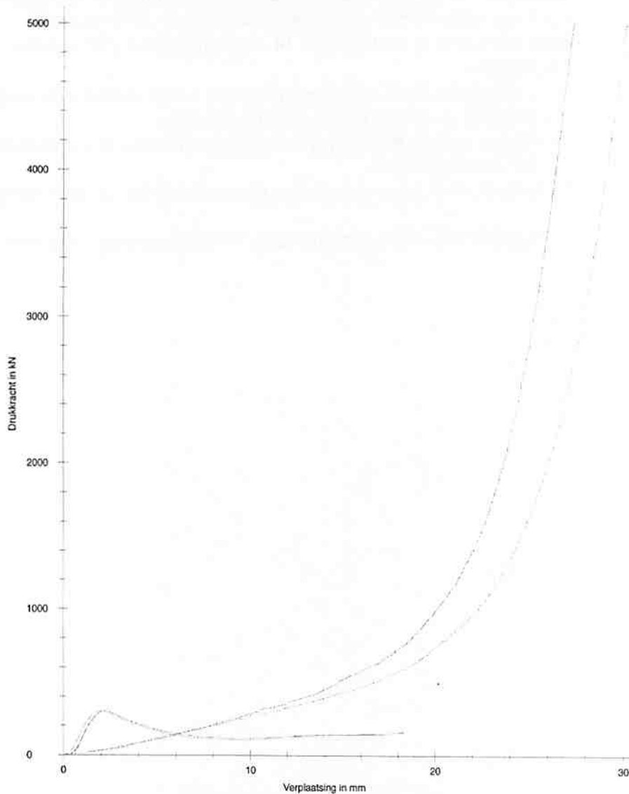
Grafiek 1. Grafische weergave beproevingsresultaten.
